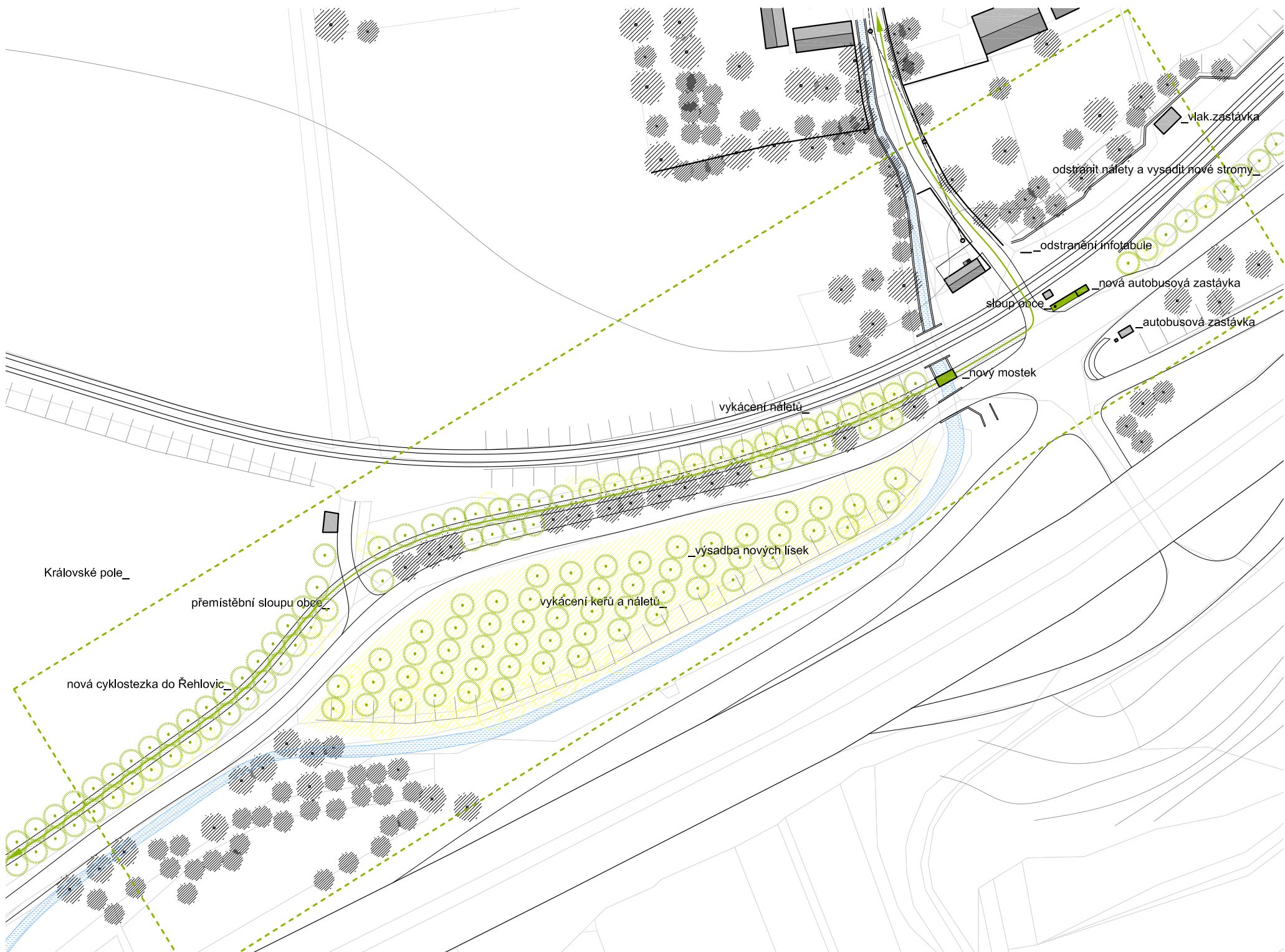
situace předprostoru královského pole a Stadice
