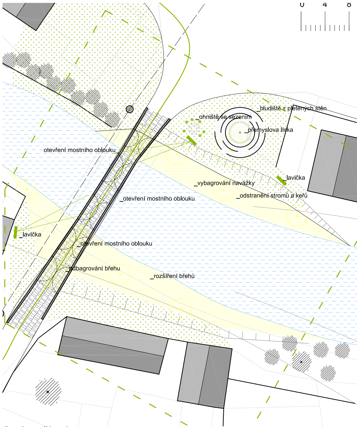
situace kamenného mostu
