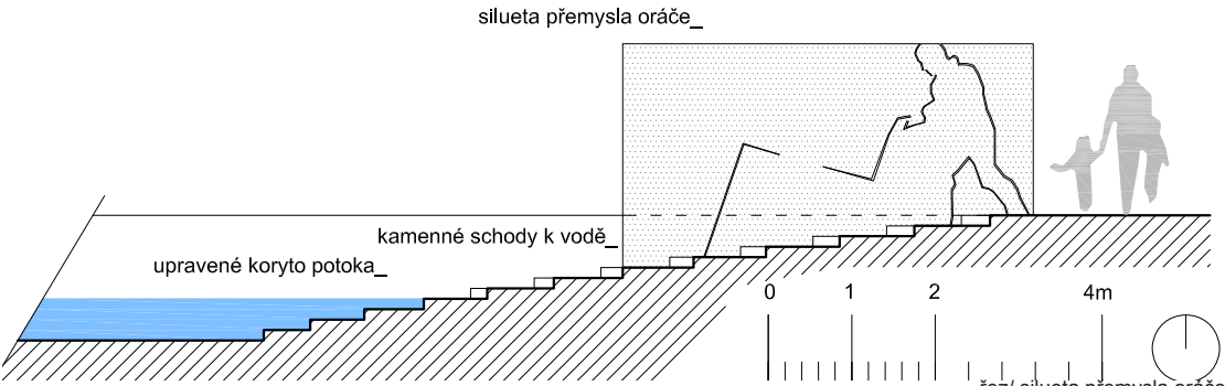
řez/ silueta přemysla oráče
