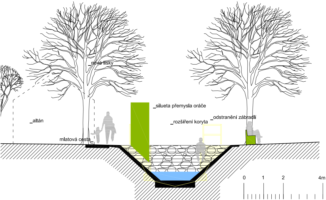
řez/ Radejčinský potok
