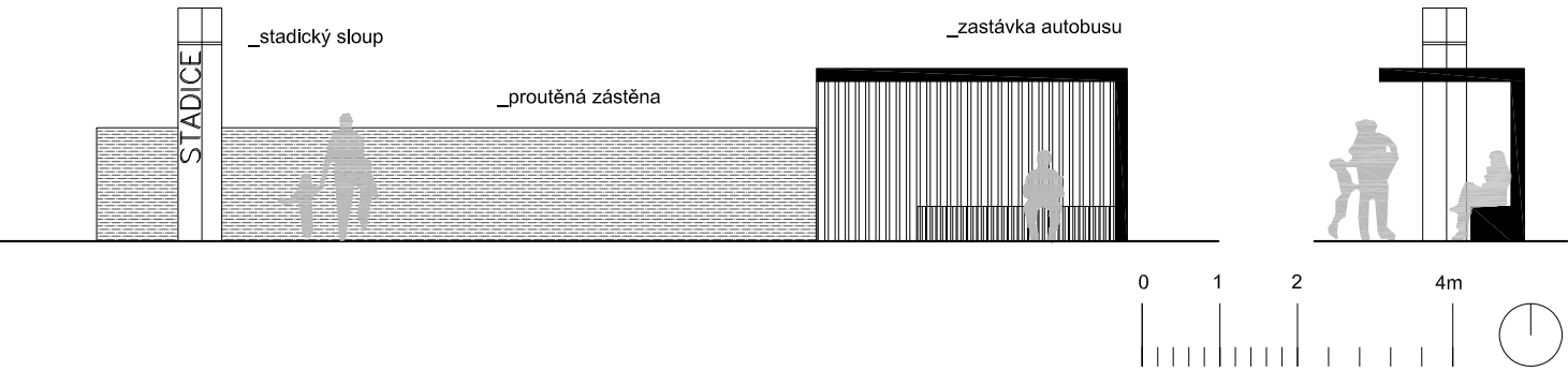
pohled a řez na autobusovou zastávku
